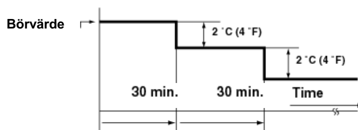
Logik nattsänkning
