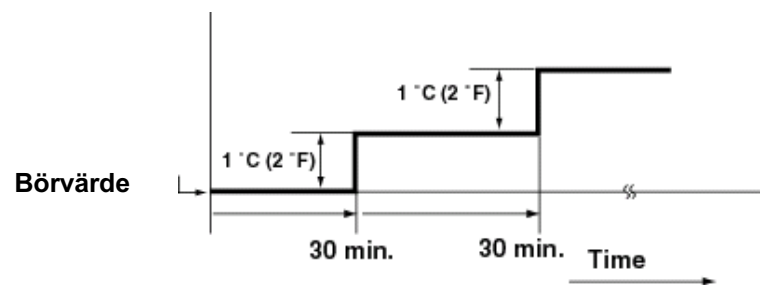
Logik nattsänkning
